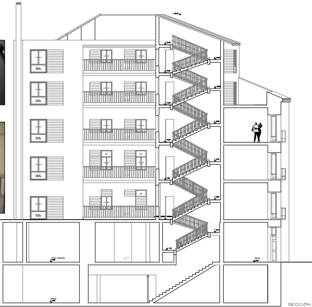
SECCIÓN LONGITUDINAL A-A
