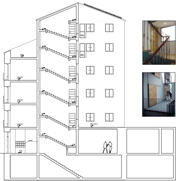
SECCIÓN LONGITUDINAL B-B
