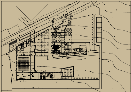
Planta general
